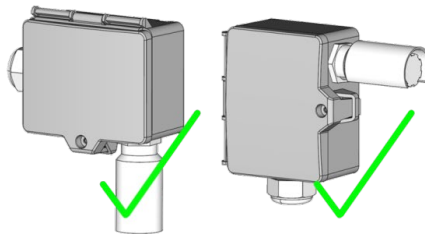
Ausrichtung korrekt
