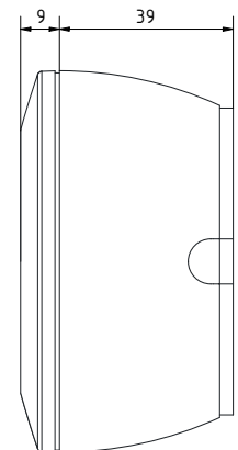
Aufputzgehäuse Surface-mounting housing
