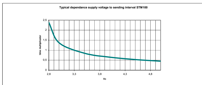
Bild: Variation der Sendeintervalle in Abhängigkeit des Energiespeichers
