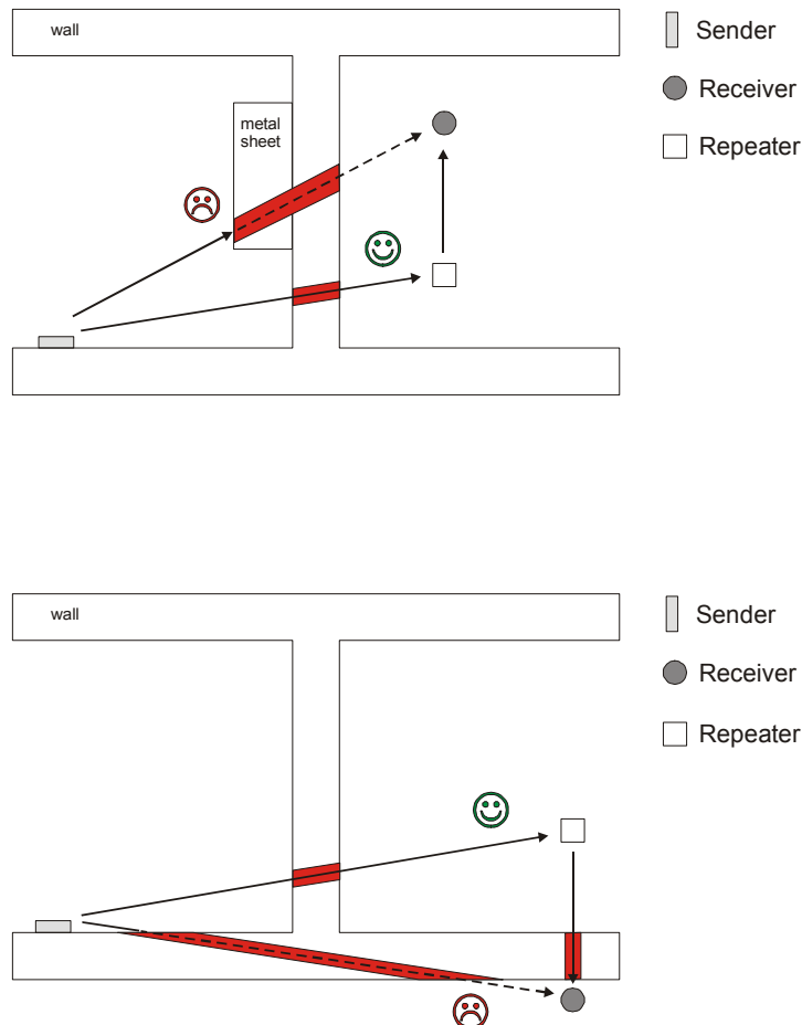
Bild: Einsatz eines Repeaters
